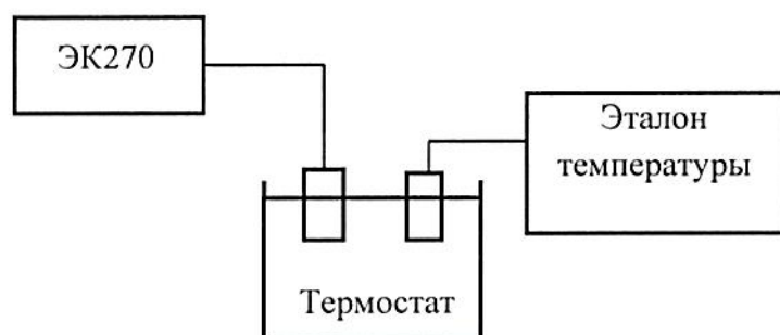
Рисунок 1 – Схема определение относительной погрешности измерения температуры Рисунок 1 (Измененная редакция, Изм. № 1)
