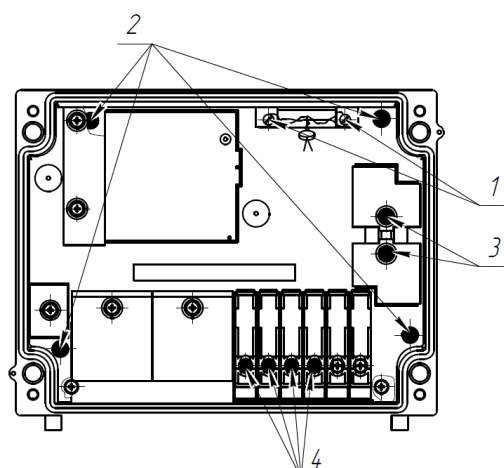
Корректор EK290
