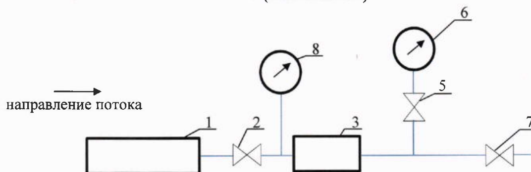
Рисунок Б.1 – Схема монтажа счетчика при проверке герметичности: 1 - компрессор; 2, 5, 7 – запорные вентиль; 3 – проверяемый счетчик; 6, 8 – манометр.
